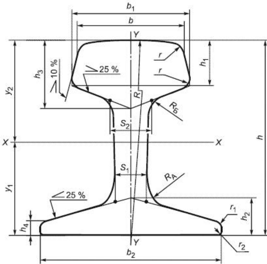
Рисунок 1 - Поперечное сечение рельсов типа КР70
