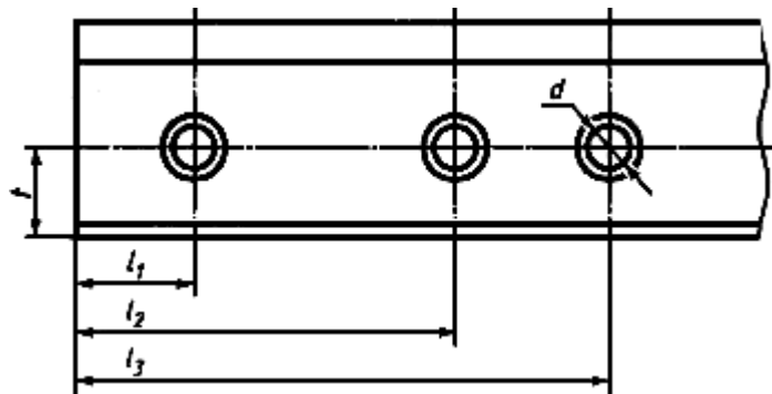
Рисунок 2 - Расположение болтовых отверстий
