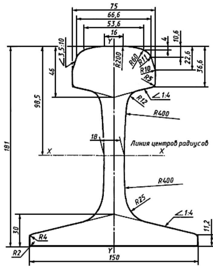
Рисунок А.3 - Рельс типа Р65К
