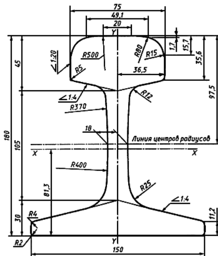
Рисунок А.2 - Рельс типа Р65
