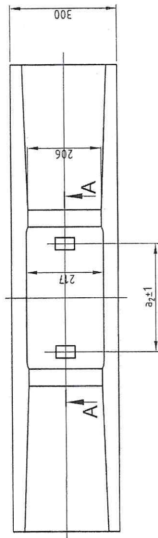
Рисунок 2. Форма и размеры полушпалы исполнения 1, для изготовления в брусковой форме
